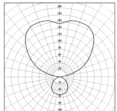
Leuchtenbetriebswirkungsgrad 65% Leuchtdichtegrenzkurve Güteklasse 1
